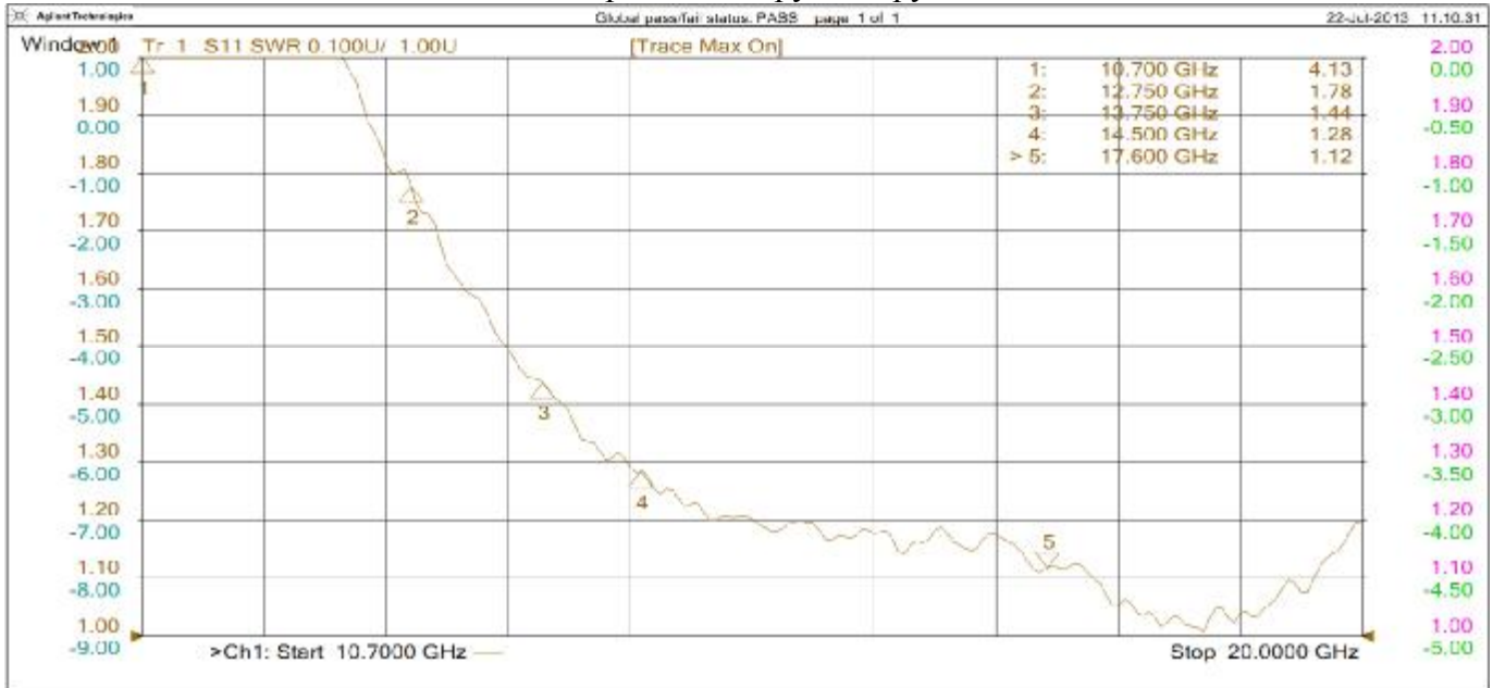
КСВН на волноводной нагрузке
